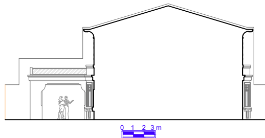
Elevação 02
