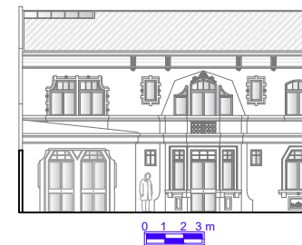
Elevação 03
