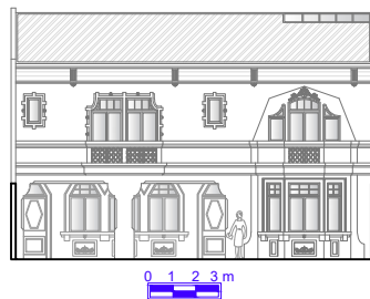
Elevação 01
